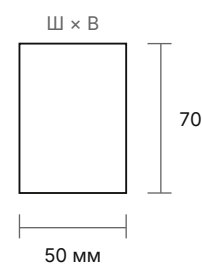
Габаритное сечение
